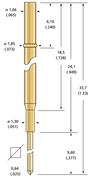
S 21.00-W Wire-Wrap-Post
