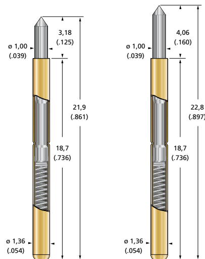
GR1.02.10.11 Spring Force 4.0 oz.
